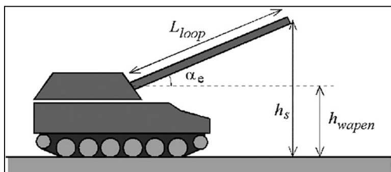
Figuur 4.1: Met de parameters h_{wapen} en L_{loop} kan de hoogte h_s van het bronpunt van de mondingssknal worden berekend voor een gegeven elevatiehoek \alpha_e . In deze afbeelding valt het bronpunt samen met de vuurmond, maar in het algemeen kan het bronpunt op enige afstand van de vuurmond liggen. L_{loop} is dan langer dan de feitelijke lengte van de loop (zie § 4.5.1).
