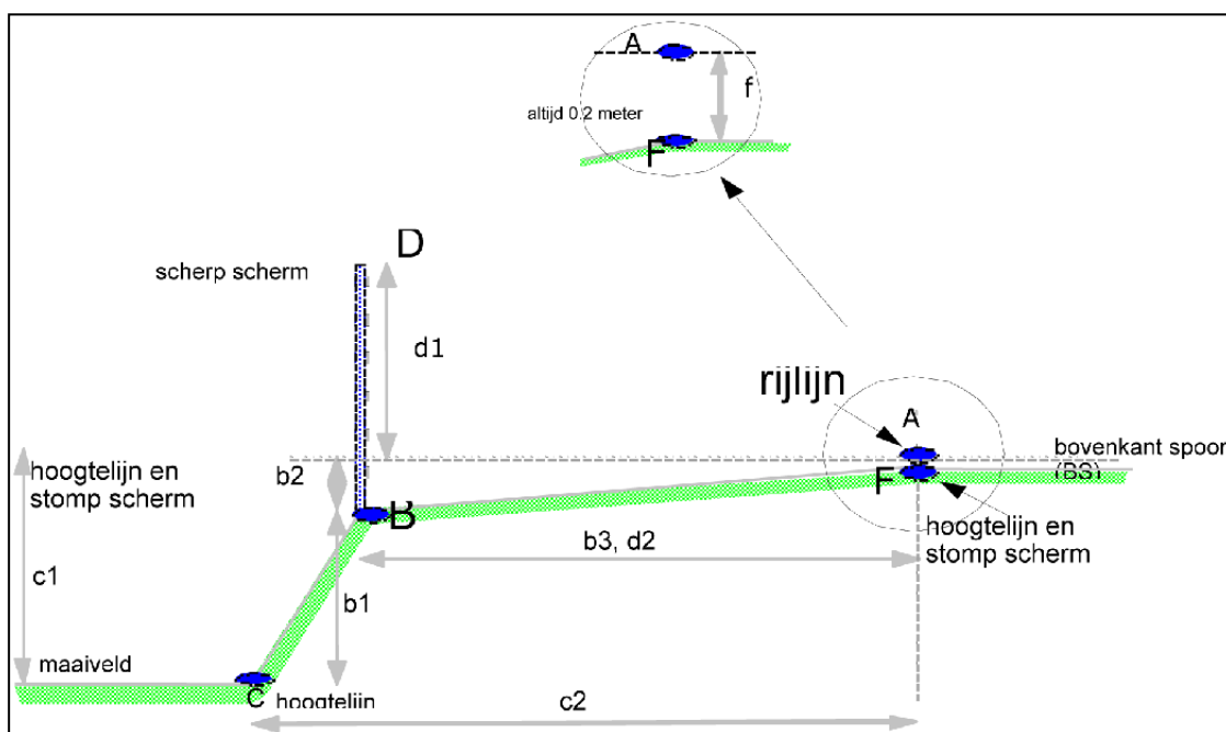
Figuur 3.4 Modelleren van de dwarsdoorsnede van een standaard talud.
