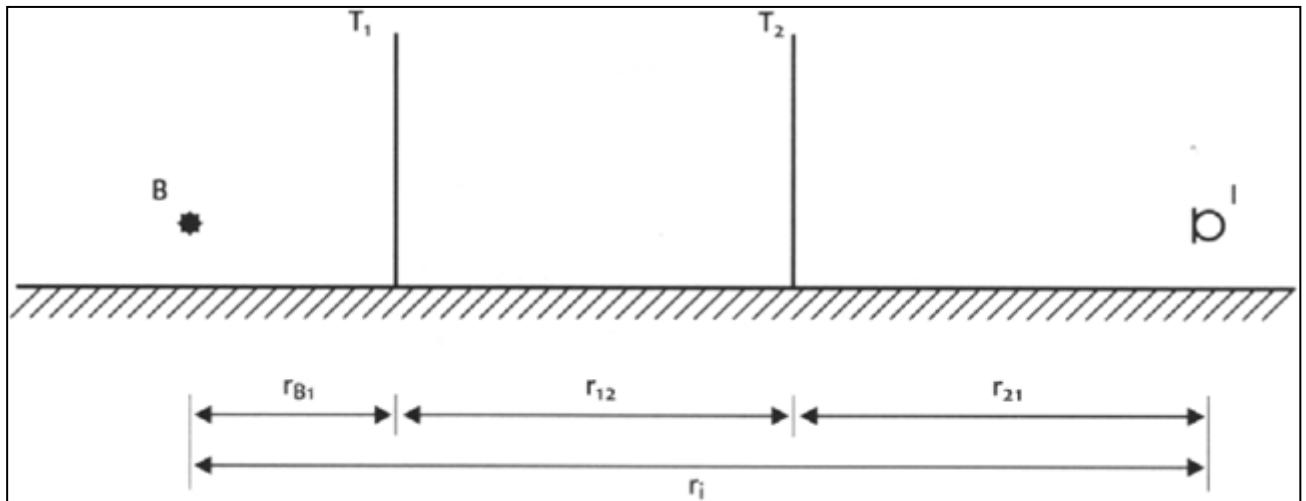
Figuur 2.7 De geometrie bij meerdere schermen tussen bron en immissiepoint.
