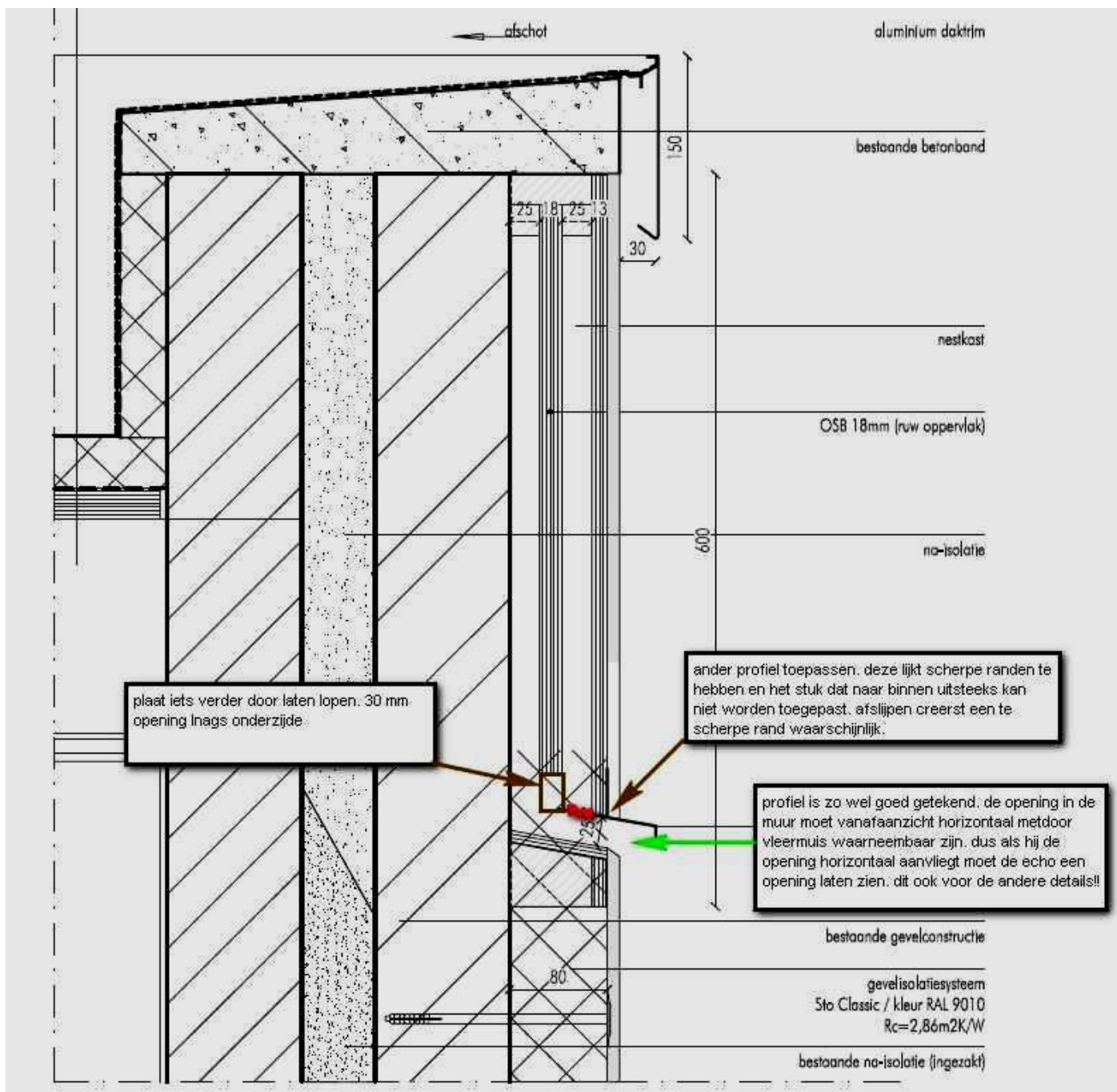
Voorbeeldtekening (dwarsdoorsnede) van een vleermuisverblijf in een aangepaste gevelrand. Het gaat hierbij om een tweelagig verblijf waarbij de binnenkant is afgewerkt met 18 mm OSB platen om te zorgen voor voldoende ruw materiaal. Hierbij dient aandacht besteed te worden aan aluminium profiel (voorkomen regeninslag) omdat dit scherpe randen heeft en dus niet mag uitsteken tot binnen het verblijf (Bron: Arcadis)
