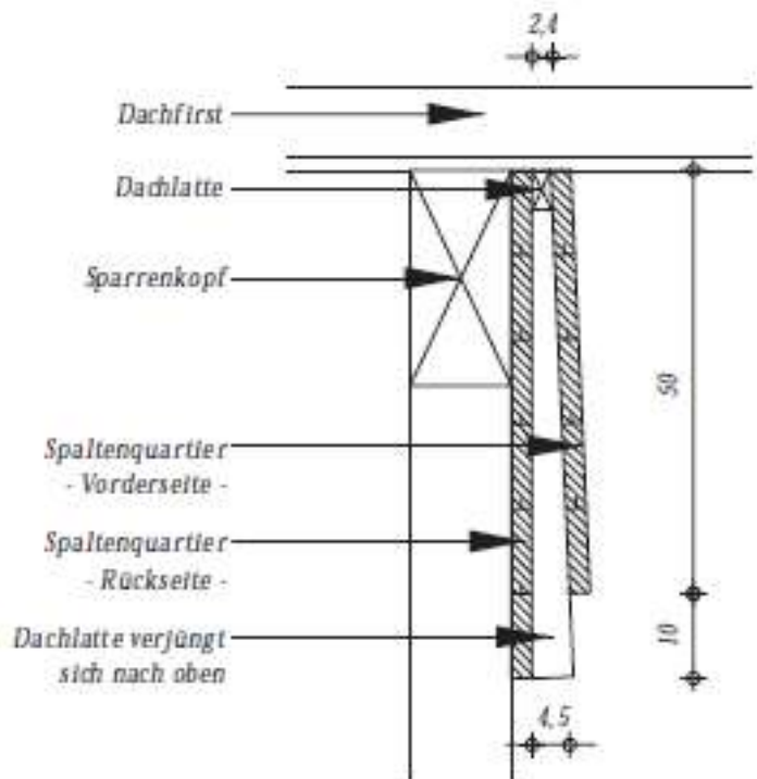
- Querschnitt - 1 : 10
