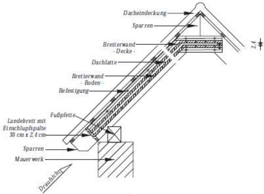
- Längsschnitt - 1:20
