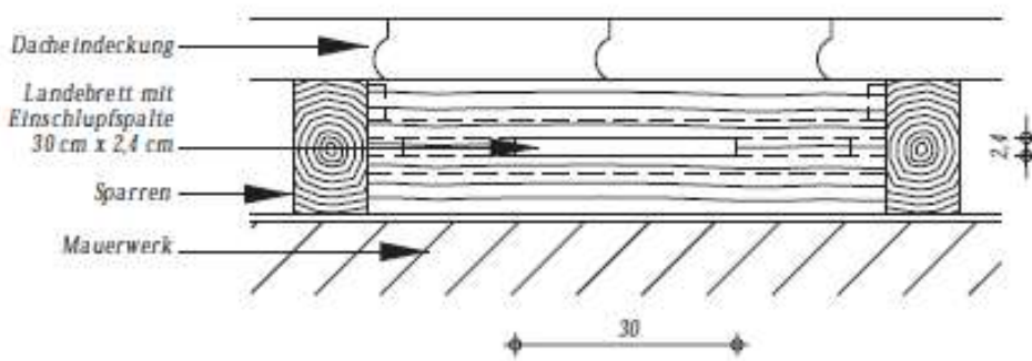
- Draufsicht - 1:10
