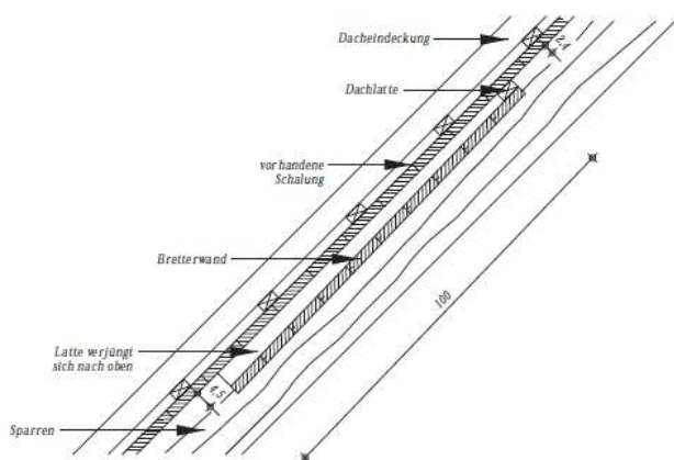
- Längsschnitt - 1 : 10
