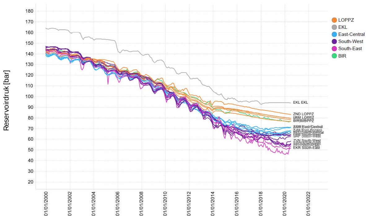
Figuur 11: Reservoir drukdaling in Groninger gasveld op basis van het gekalibreerde Groningen reservoirmodel. Merk op dat de druk in de cluster Loppersum (LOPPZ) ook bij verminderde en stilgelegde productie daalt.
