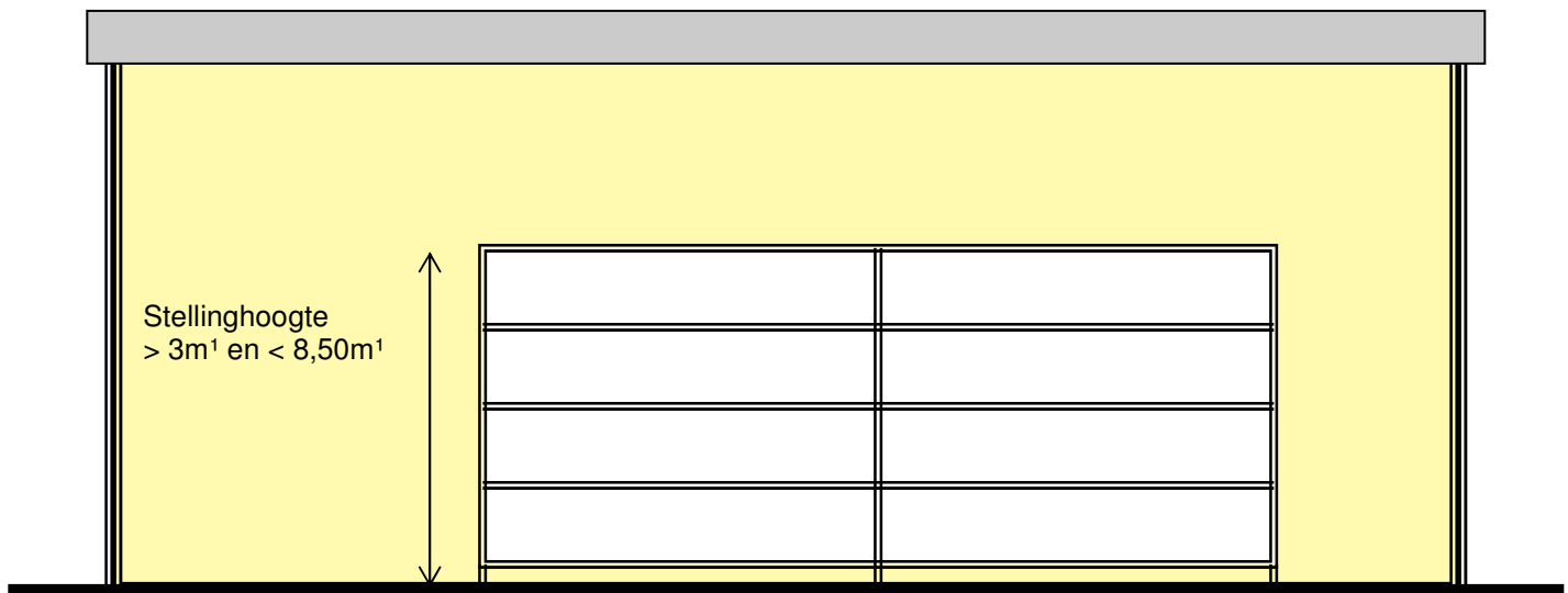
Doorsnede gebouw
