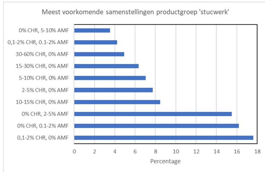
Figuur 6: Meest frequent voorkomende samenstellingen van productgroepen binnen hoofdproductgroep 'licht-gebonden' op basis van SMA-rt-uitdraaien over de periode 2014-2016
