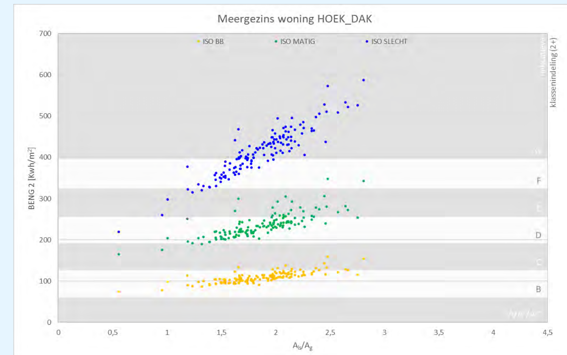
figuur 17: Spreiding A w /A g en BENG 2 meergezinswoning HOEK_DAK
