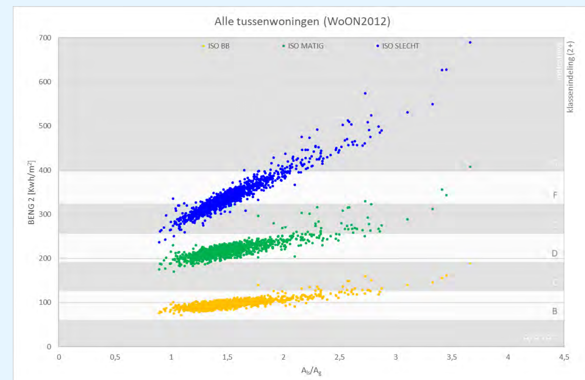
figuur 18: Spreiding A w /A g en BENG 2 tussenwoning
